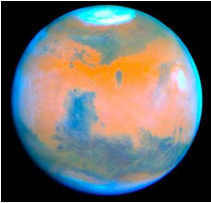
Planet Mars
