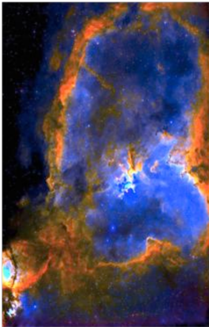
Heart nebula
